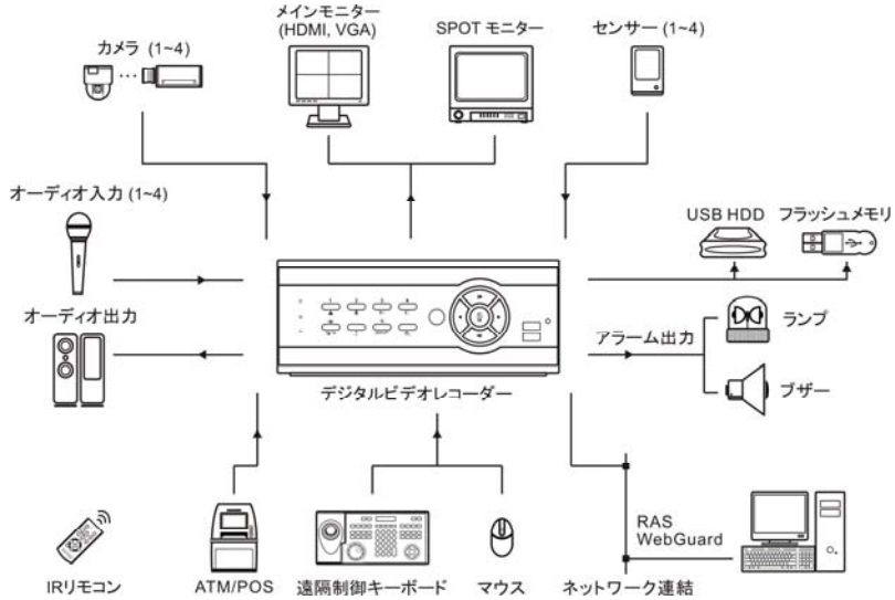
図 1: サンプル構成図
