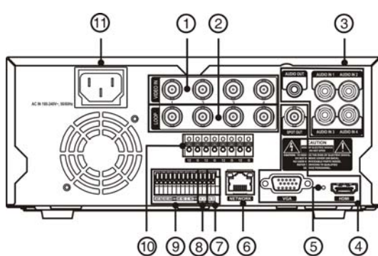
図2: DVR背面パネル
