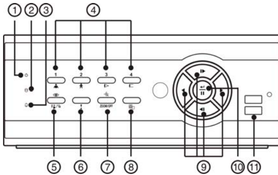
図3: DVR前面パネル
