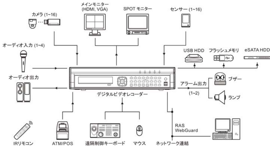
図 1: サンプル構成図
