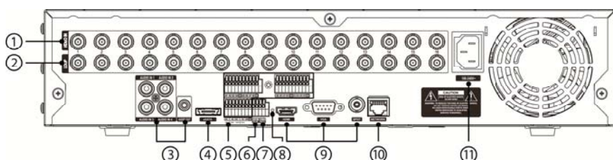
図2: 16チャンネルDVR背面パネル
