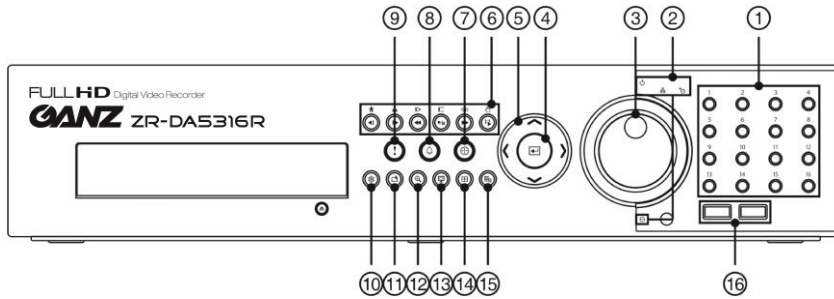
図3: DVR前面パネル
