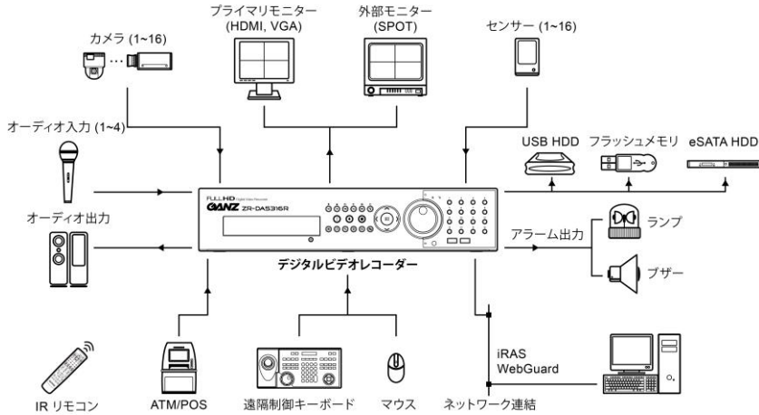
図1: サンプル構成図
