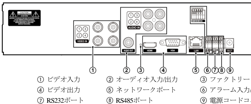
図 2: DVR背面パネル
